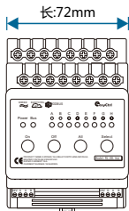
图2. 尺寸图-正面
