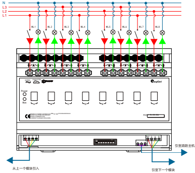
图8.产品接线图
