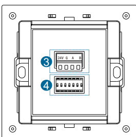
图11.面板背面
