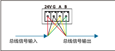
图13.总线接口接线图
