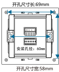
图14.安装孔位图
