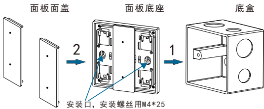
图15.面板
