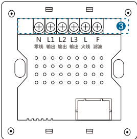
图7.面板背部
