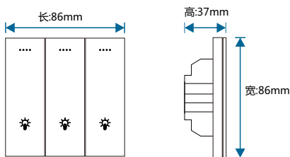
图9.尺寸图-正面
