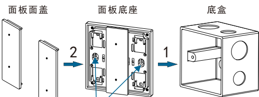
图12.面板
