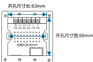
图11.安装孔位图
