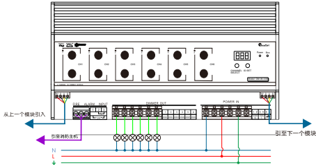
图9.产品接线图
