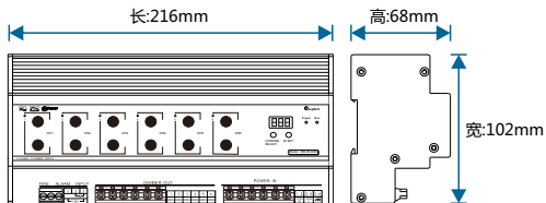
图2. 尺寸图-正面
