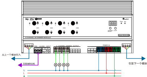
图9.产品接线图
