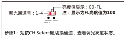
图5. 调光亮度状态查询说明
