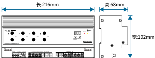
图2. 尺寸图-正面
