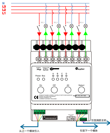
图8.产品接线图
