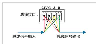
图7.总线接口接线图
