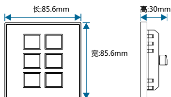
图8.尺寸图-正面
