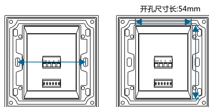
图10.安装孔位图
