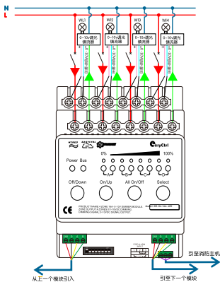
图8.产品接线图
