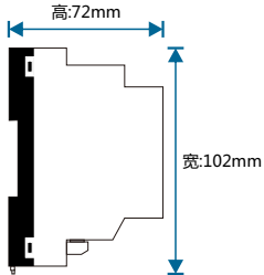
图3. 尺寸图-侧面
